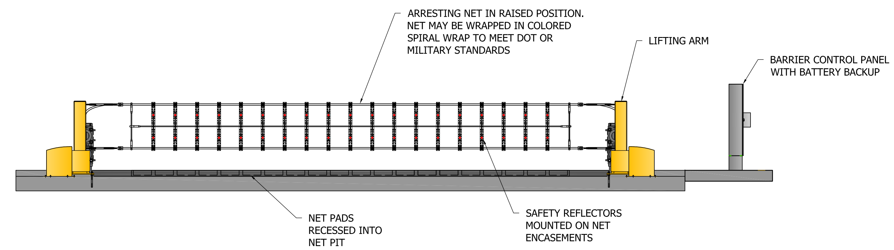
A-1 - ELEVATION VIEW SCALE: 1/4" = 1'-0"
